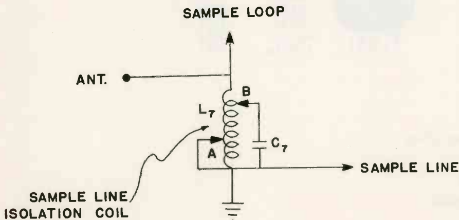
Fig. 3. De-Tuning Net.
